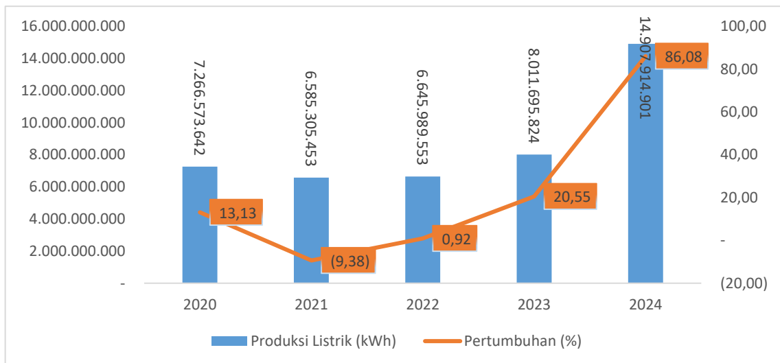
Gambar 2. 41 Produksi Listrik di Provinsi Sumatera Selatan (KWh), 2020-2024
