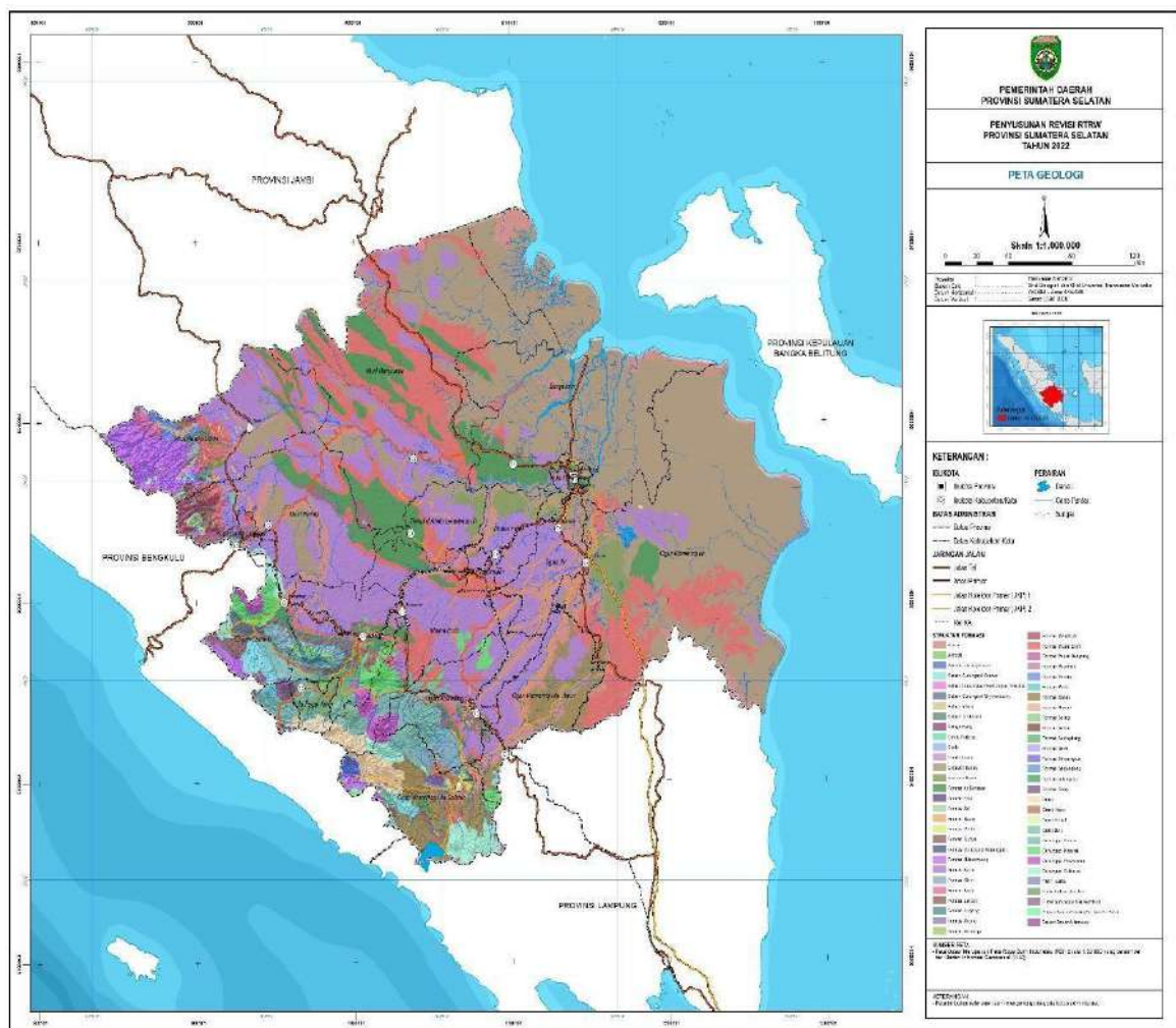
Gambar 2. 6 Peta Geologi Provinsi Sumatera Selatan
