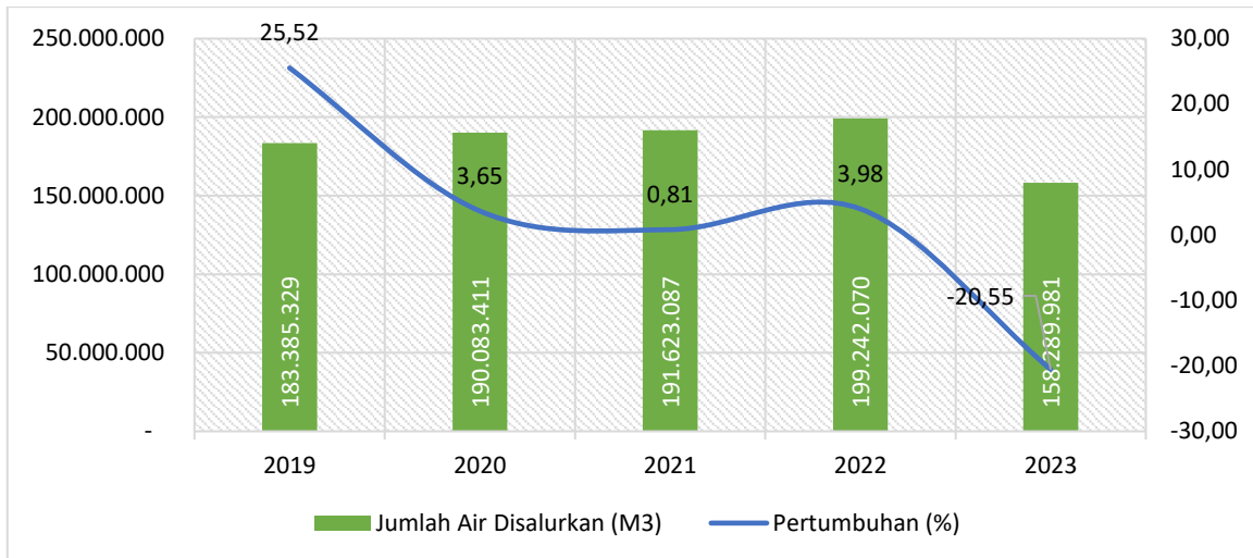
Gambar 2. 36 Jumlah Air Disalurkan di Provinsi Sumatera Selatan (m 3 ), 2019-2023
