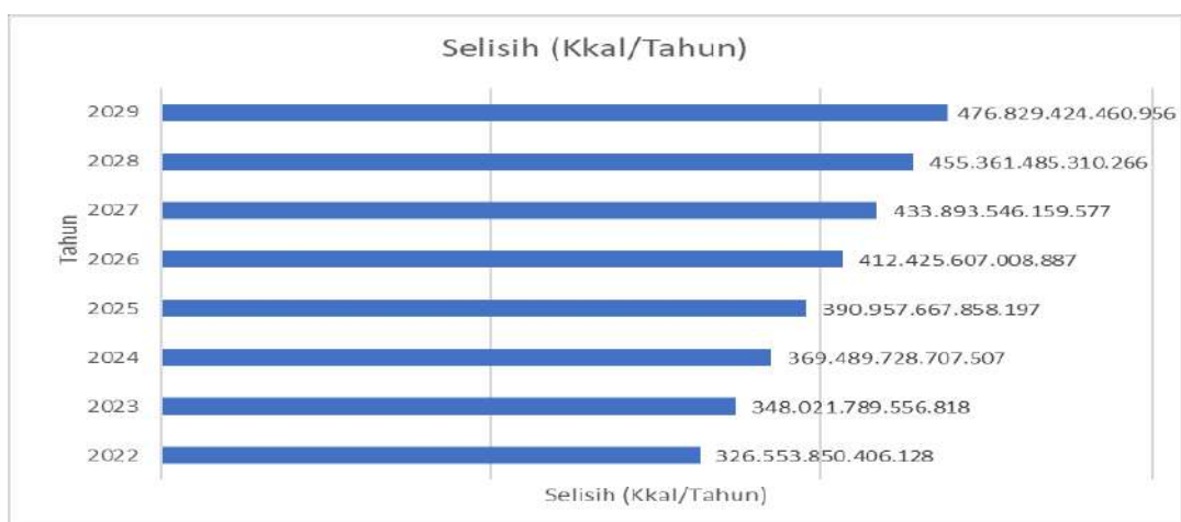
Gambar 2. 39 Grafik Selisih/Cadangan Pangan Provinsi Sumatera Selatan
