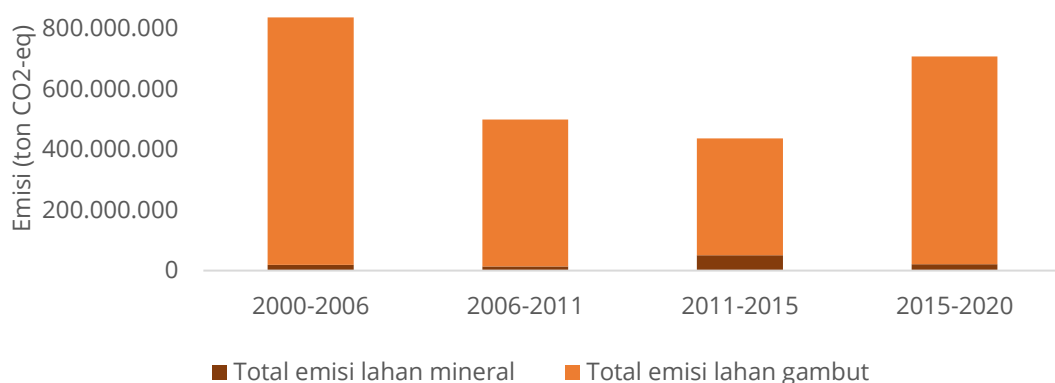
Gambar 2. 16 Emisi Berbasis Lahan Historis Sumatera Selatan Tahun 2000-2020
