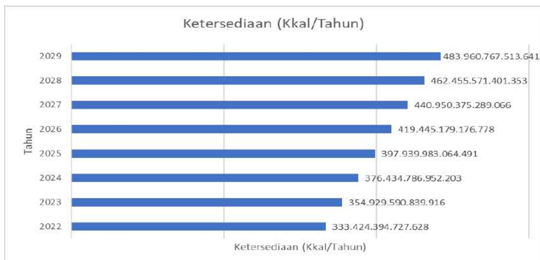
Gambar 2. 38 Grafik Ketersediaan Pangan Provinsi Sumatera Selatan
