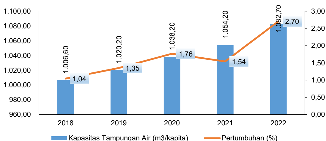
Gambar 2. 35 Kapasitas Tampung Air di Provinsi Sumatera Selatan (m 3 /kapita), 2018-2022
