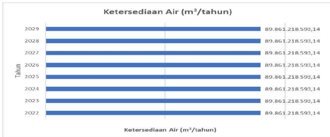
Gambar 2. 27 Ketersediaan Air Provinsi Sumatera Selatan
